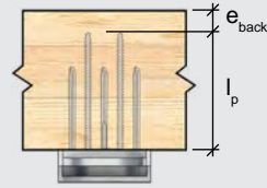
Unhoused
